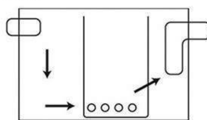
Вариант жироуловителя с камерой посередине
